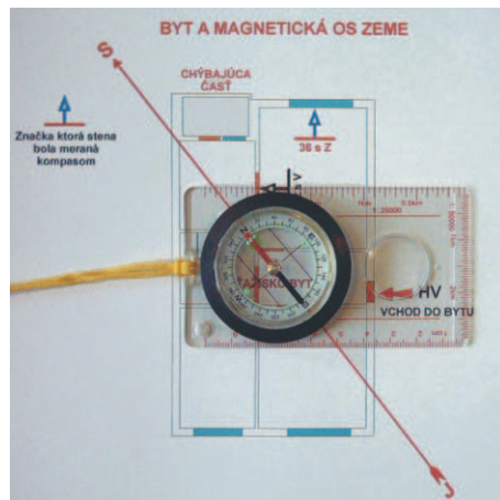
Tu vidíme, ako položiť kompas so zameranou magnetickej osou zeme na pôdorys analyzovaného objektu.
